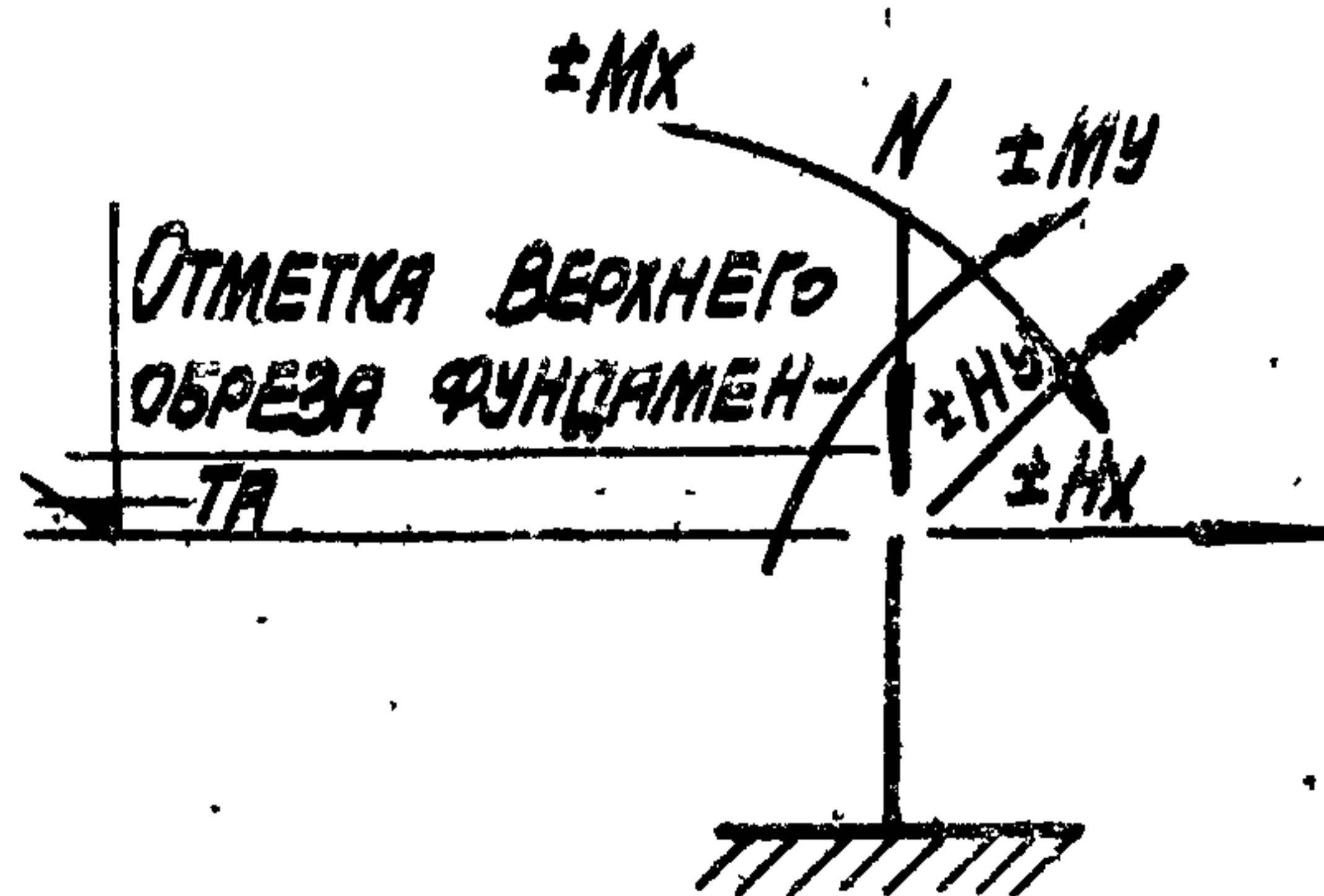
СХЕМА НАГРУЗОК НА ФУНДАМЕНТ
